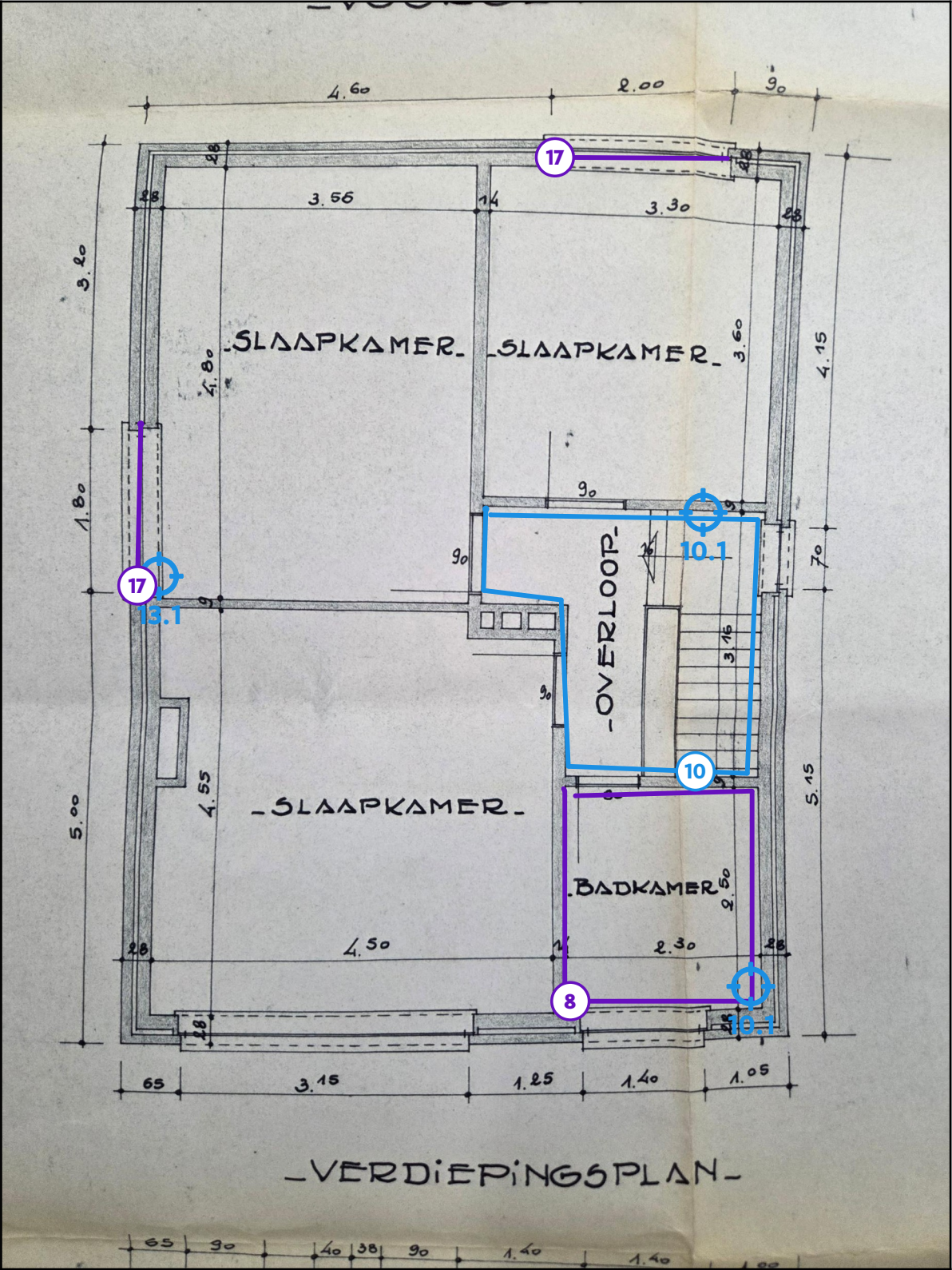
Legende van plan 1.3: Verdiepingsplan
